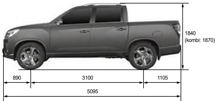
Oldalnézet
