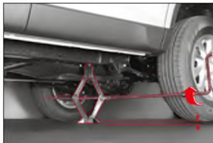
Emelési pontok
