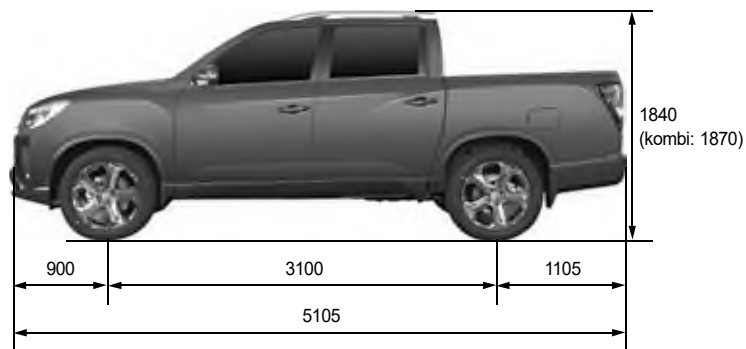
Oldalnézet
